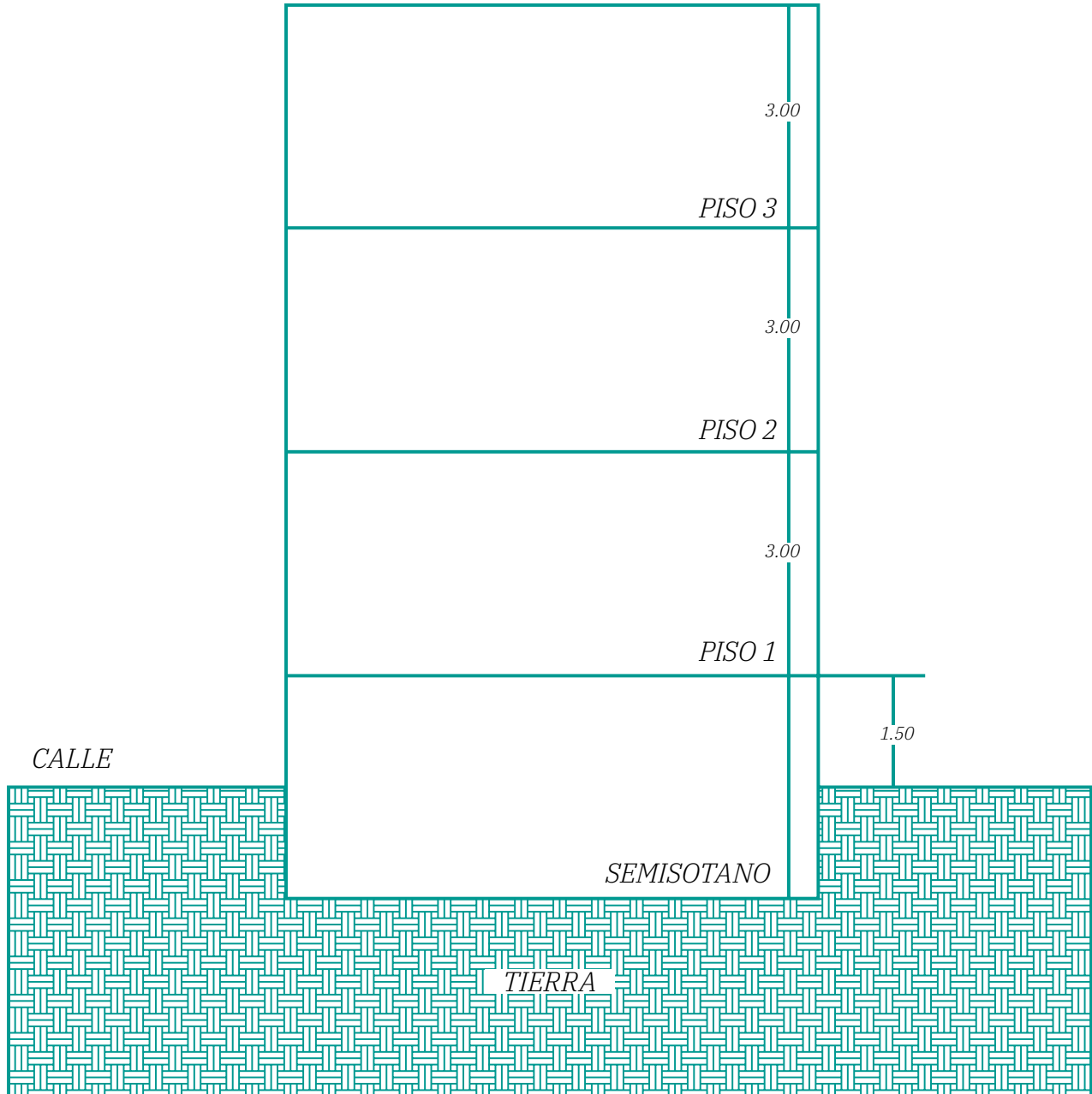
SECCIÓN EDIFICIO 3 PISOS CON SEMISOTANO ESCALA 1:100
